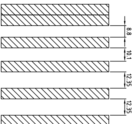
30m-Gleisjoch
