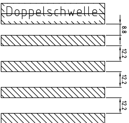
15m-Gleisjoch
