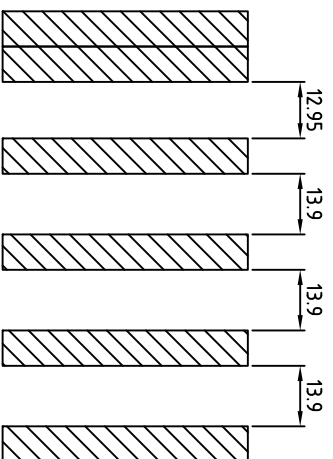
15m-Gleisjoch 1e
